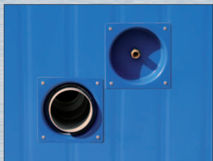
Wateraansluiting in de muur verzonken
